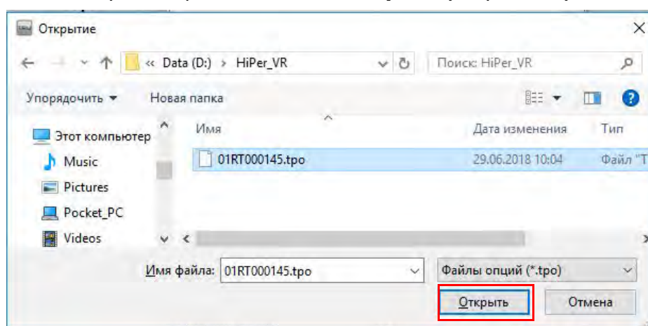
Рисунок 5-7: Загрузка OAF
